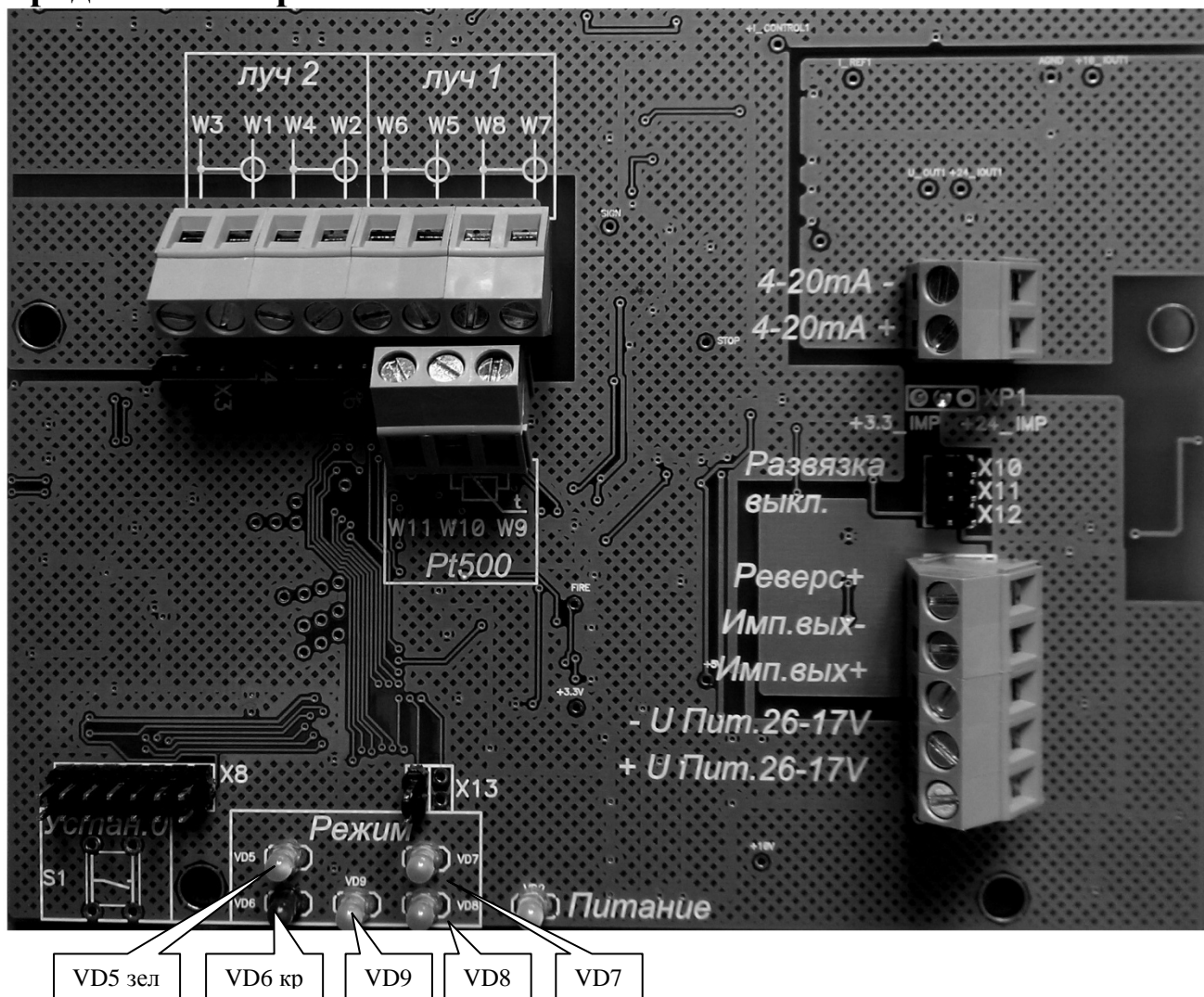
Рисунок Б.2 Вид клемм внешних подключений и диагностических светодиодов двухлучевого расходомера.
